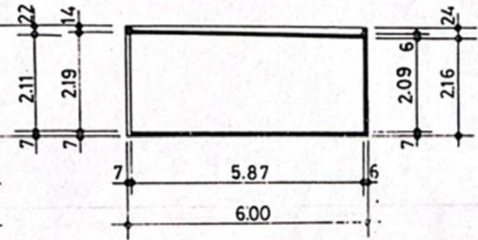
LÄNGSSCHNITT
