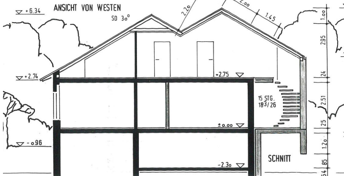
Bauantragsplan Erweiterung Wohnhaus (1991, Ausschnitt, ohne Maßstab): Ansicht Ost, West, Schnitt
