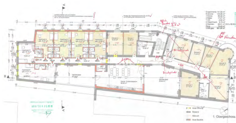
Grundriss 1.OG, Wohnflächen
