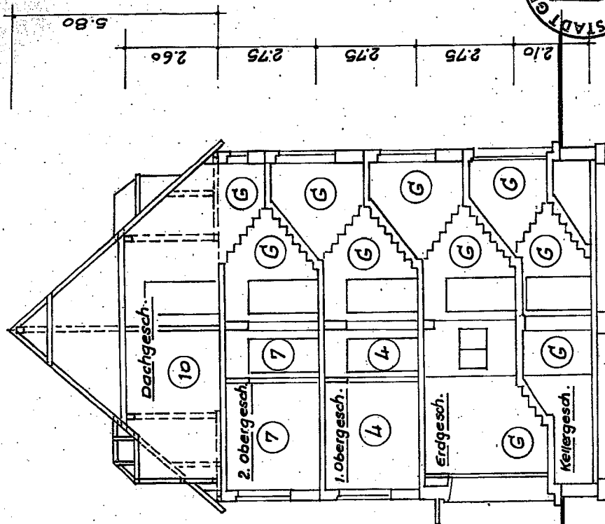
Schnitt 1-1
