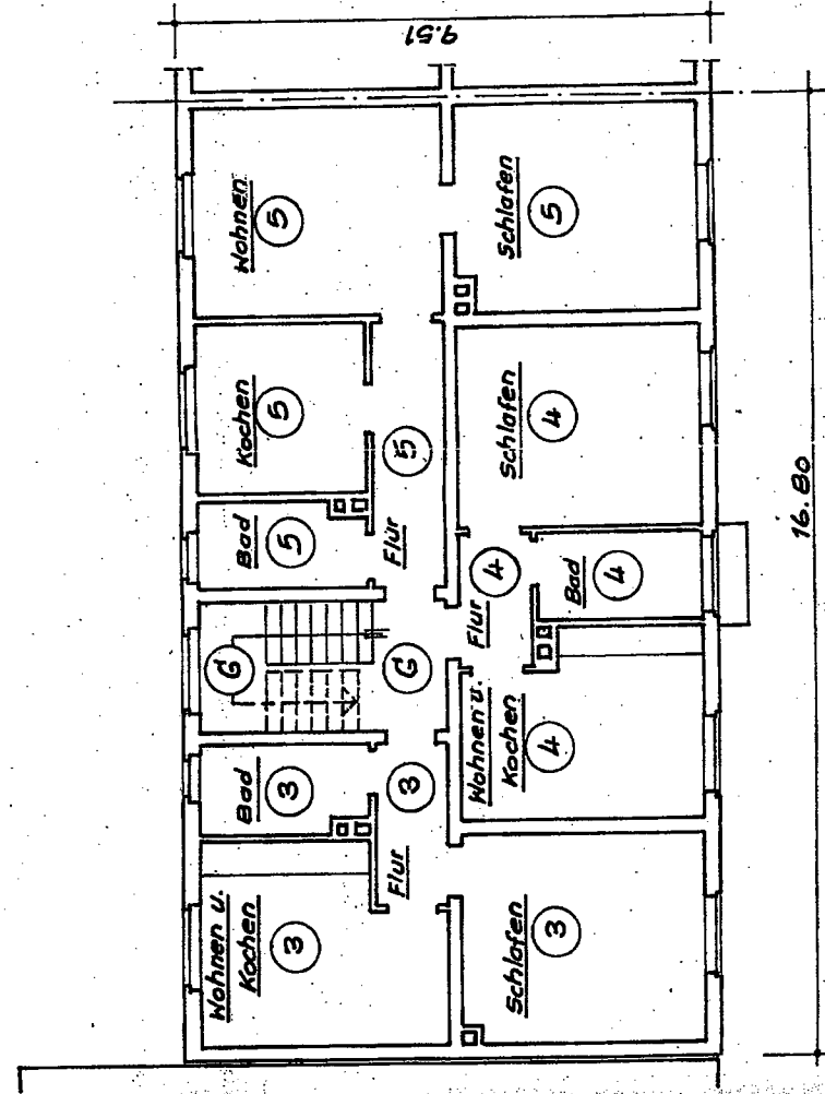
1. Obergeschoß
