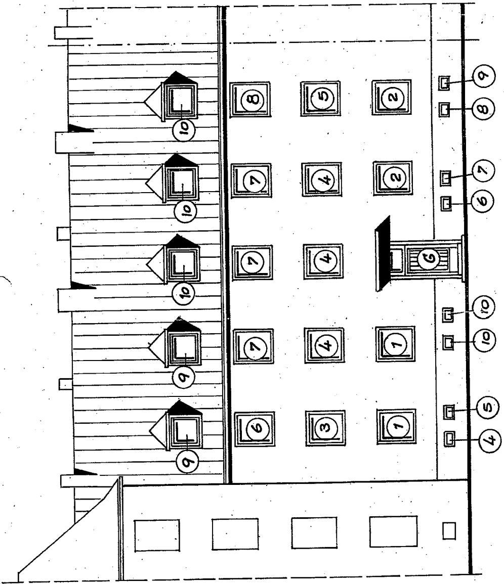
Straßenansicht
