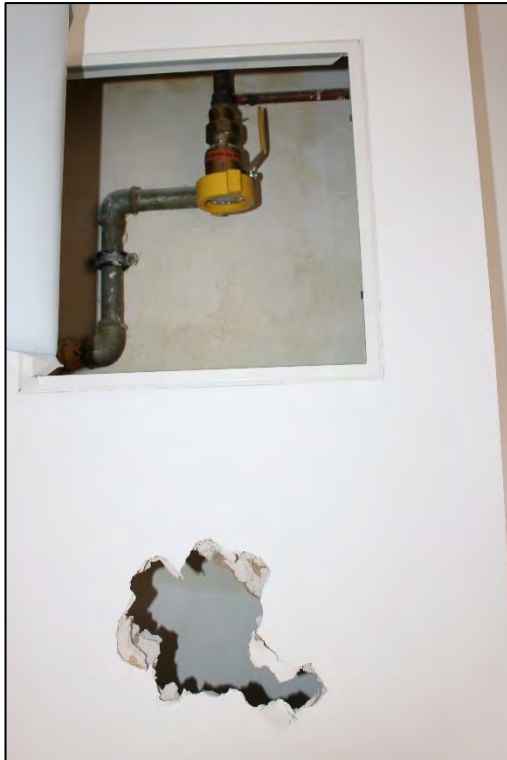
Foto Nr. 65: Dachgeschoss, WE Nr. 5, Diele / Gasanschluss
