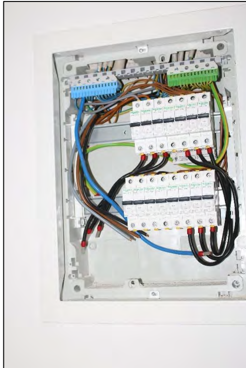
Foto Nr. 59: Dachgeschoss, WE Nr. 5, Flur rechts, Elektrounterverteilung
