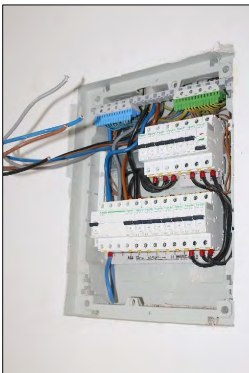
Foto Nr. 54: Dachgeschoss, WE Nr. 5, Elektrounterverteilung, Diele links
