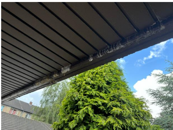
Bild 11: Abplatzungen
