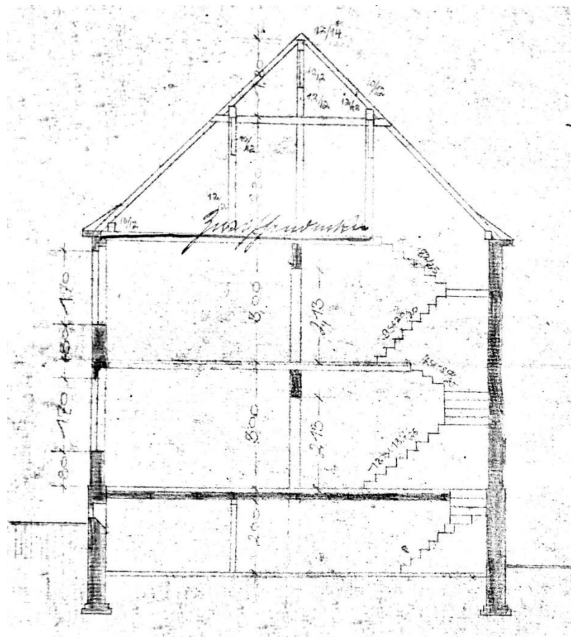
Schnitt
