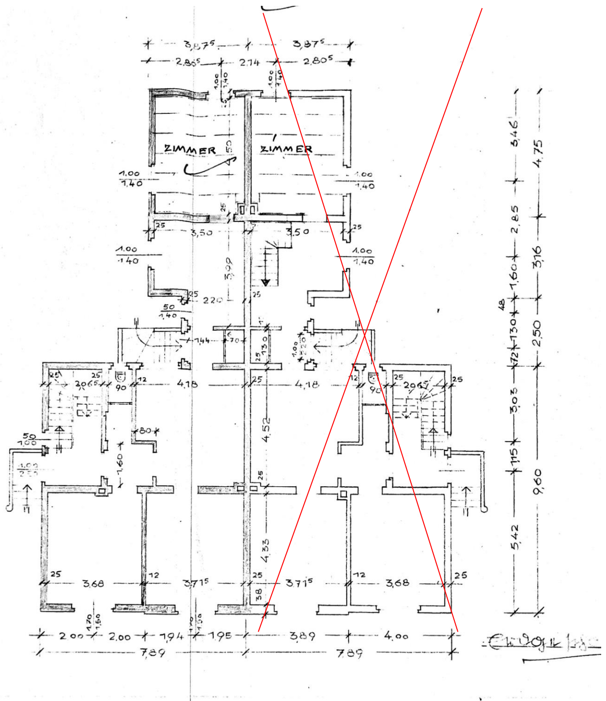
Erdgeschoss
