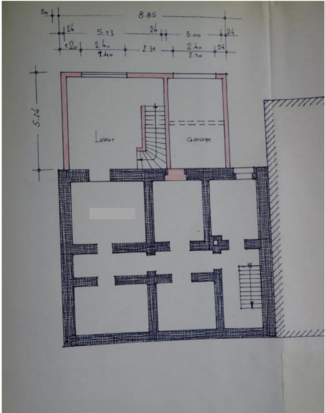
Kellergeschoss lt. Bauakte
