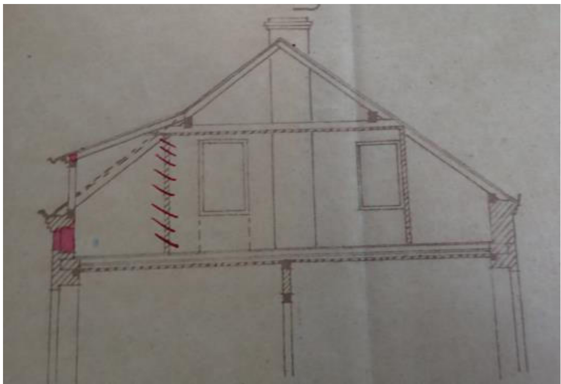
Dachgeschoss lt. Bauakte
