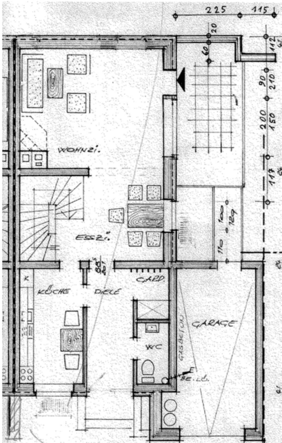
Erdgeschoss
