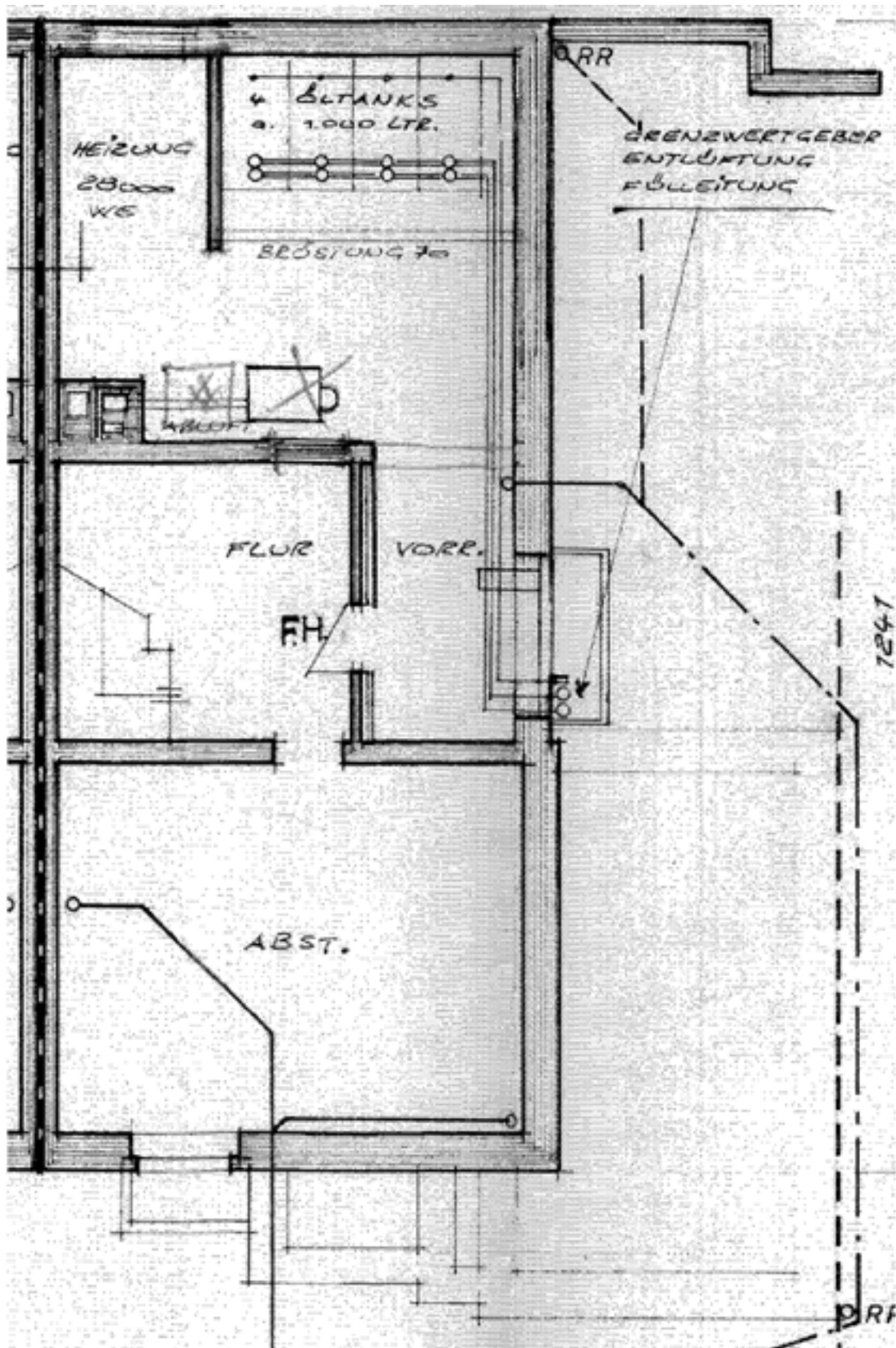
Kellergeschoss
