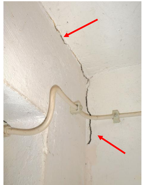
Erdgeschoss: Übergangsbereich vom Wohnen zum Abstellraum
