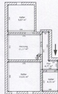
Grundriss Keller
