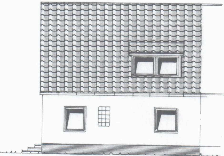
Nordansicht. _
