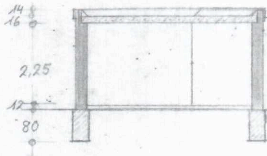
Querschnitt
