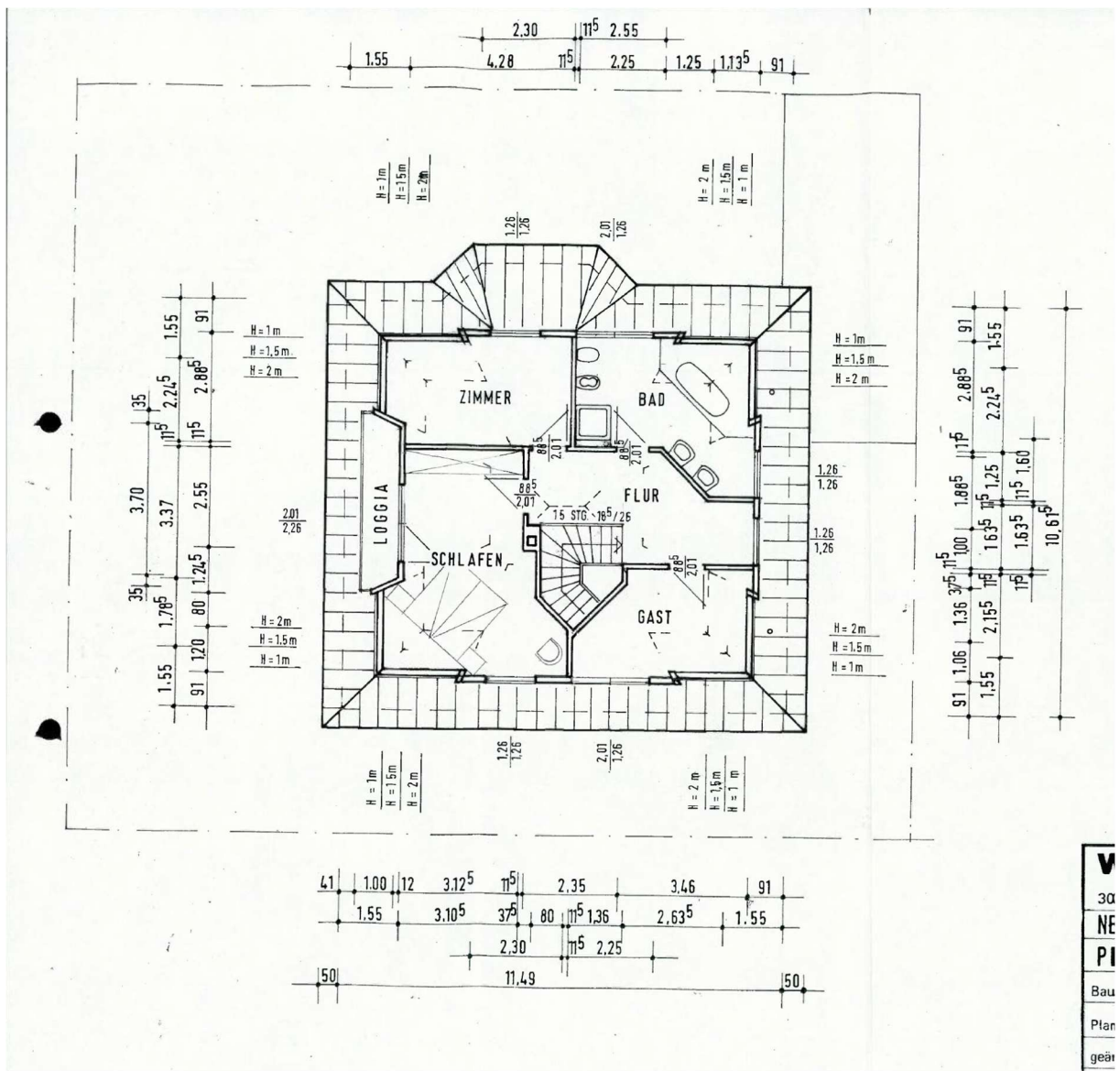
Grundriss Dachgeschoss
