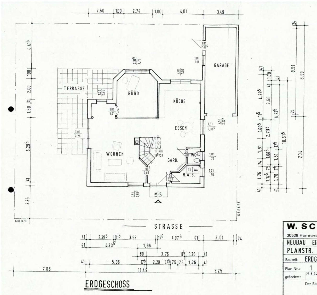
Grundriss Erdgeschoss
