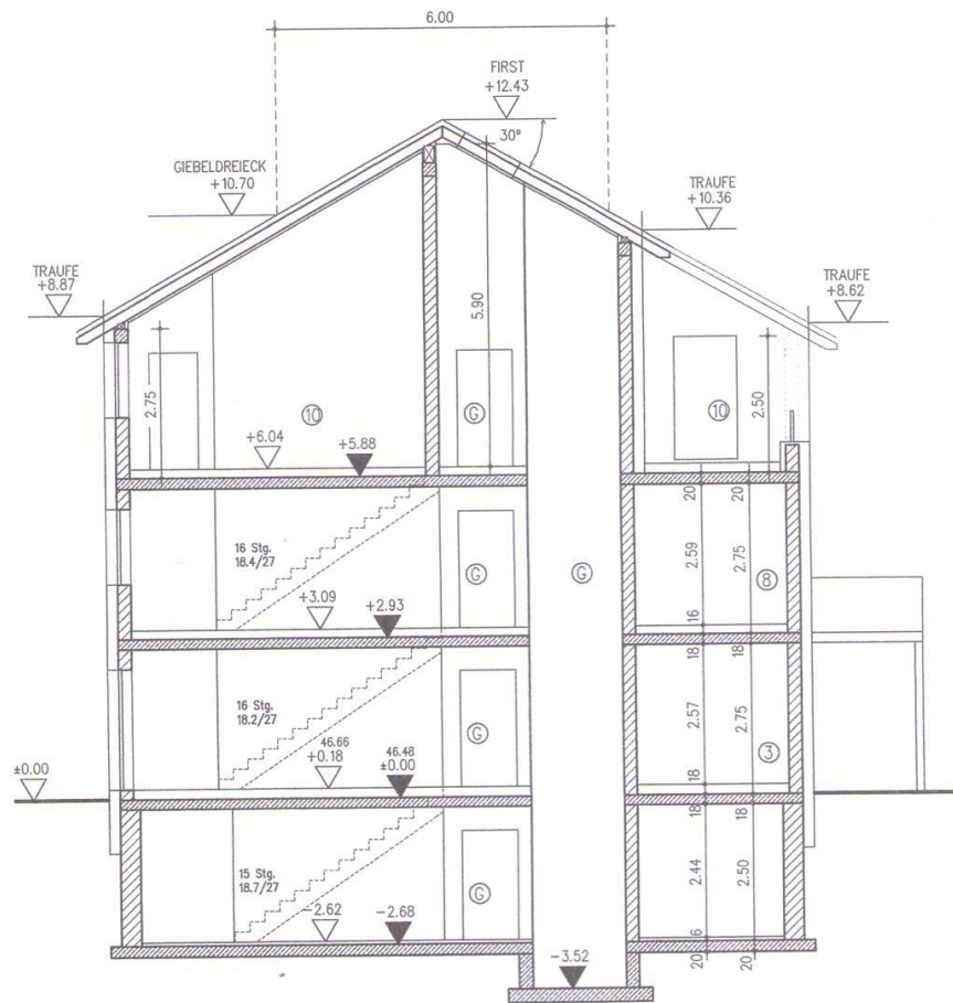
Schnitt A-A
