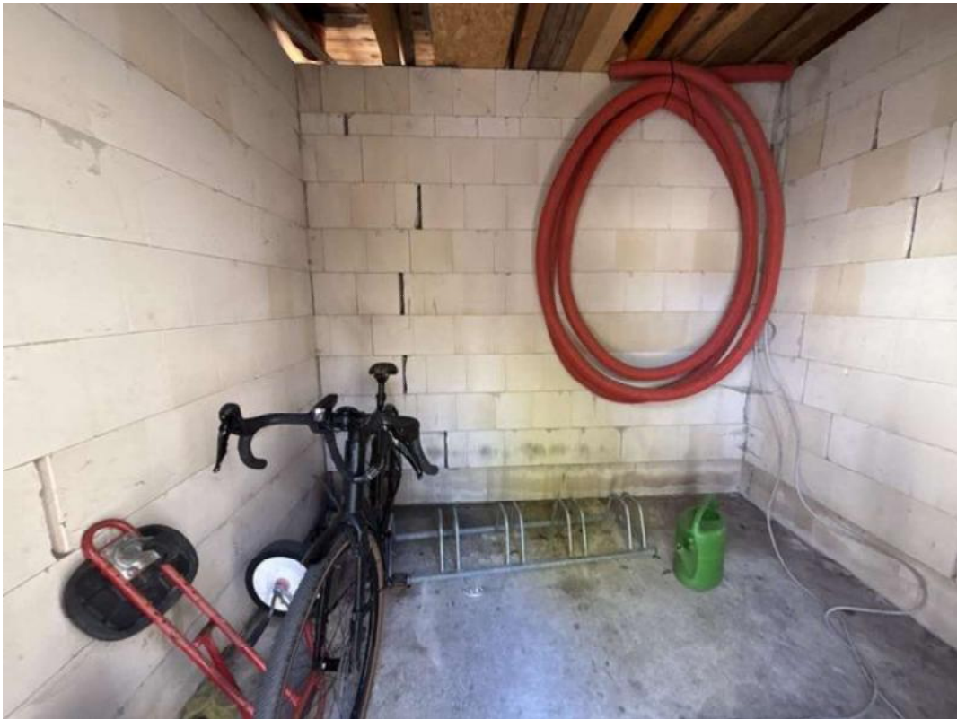
Bild 67 - Nebengebäude, Feuchtigkeitsschaden, Risse Mauerwerk
