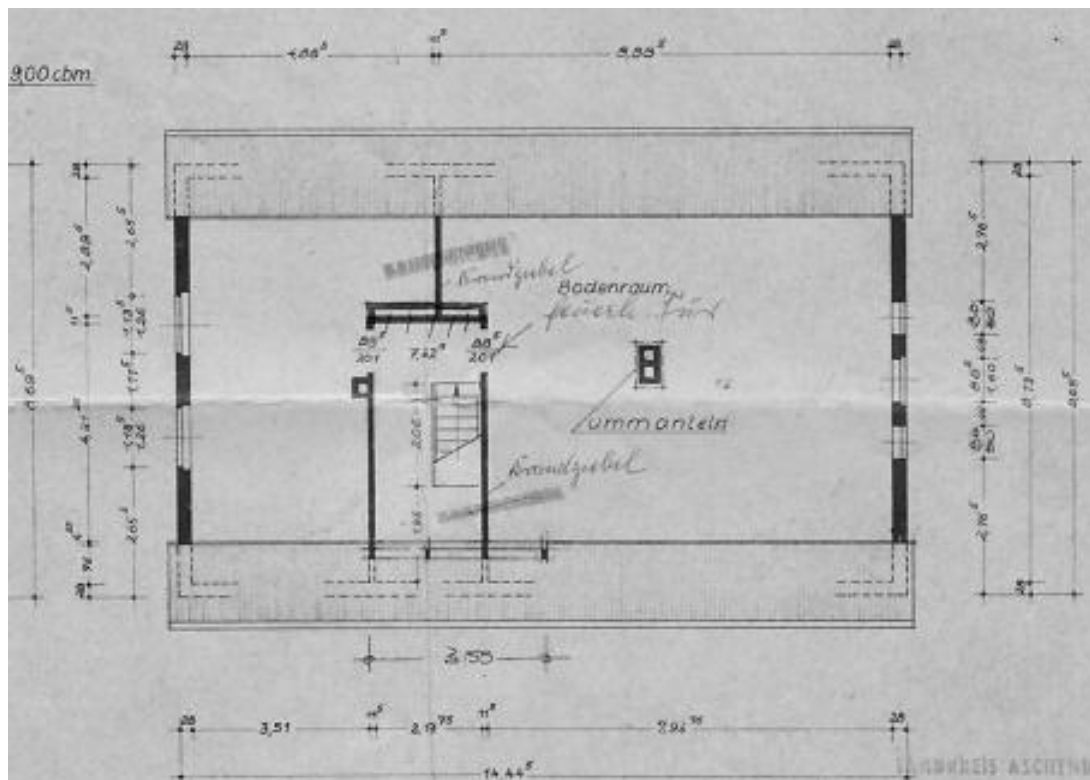
Grundriss DG aus dem Jahre 1956
