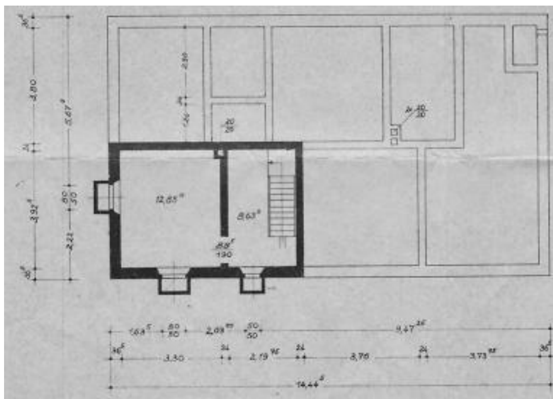
Grundriss Keller aus dem Jahre 1956
