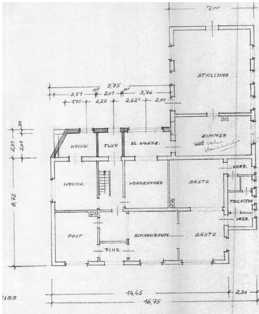
Grundriss EG aus dem Jahre 1970
