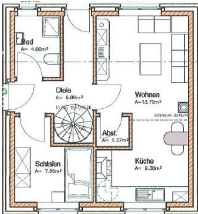
Grundriss – Erdgeschoss
