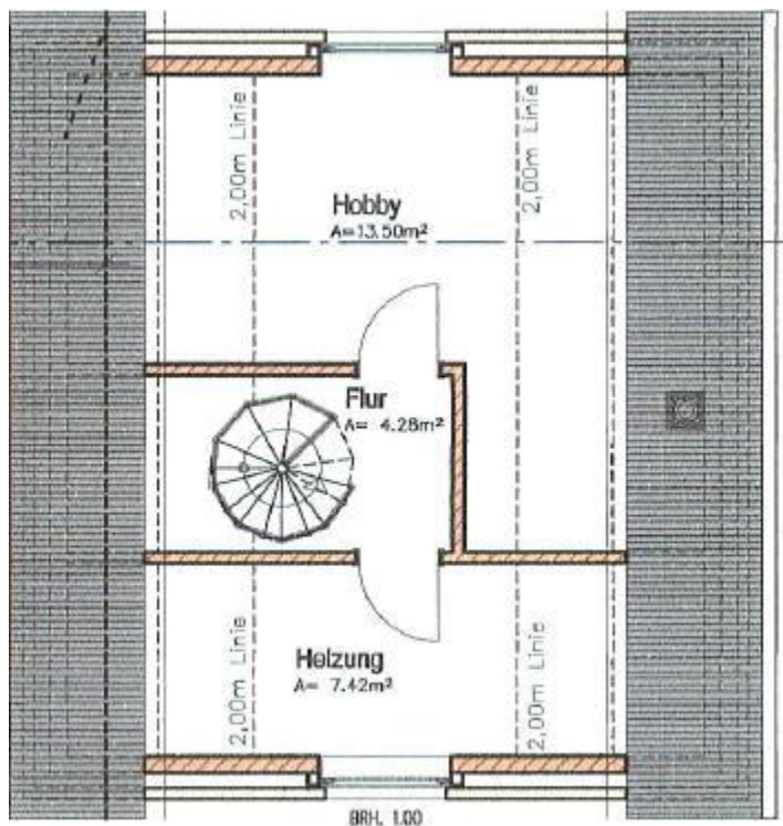
Grundriss – Dachgeschoss
