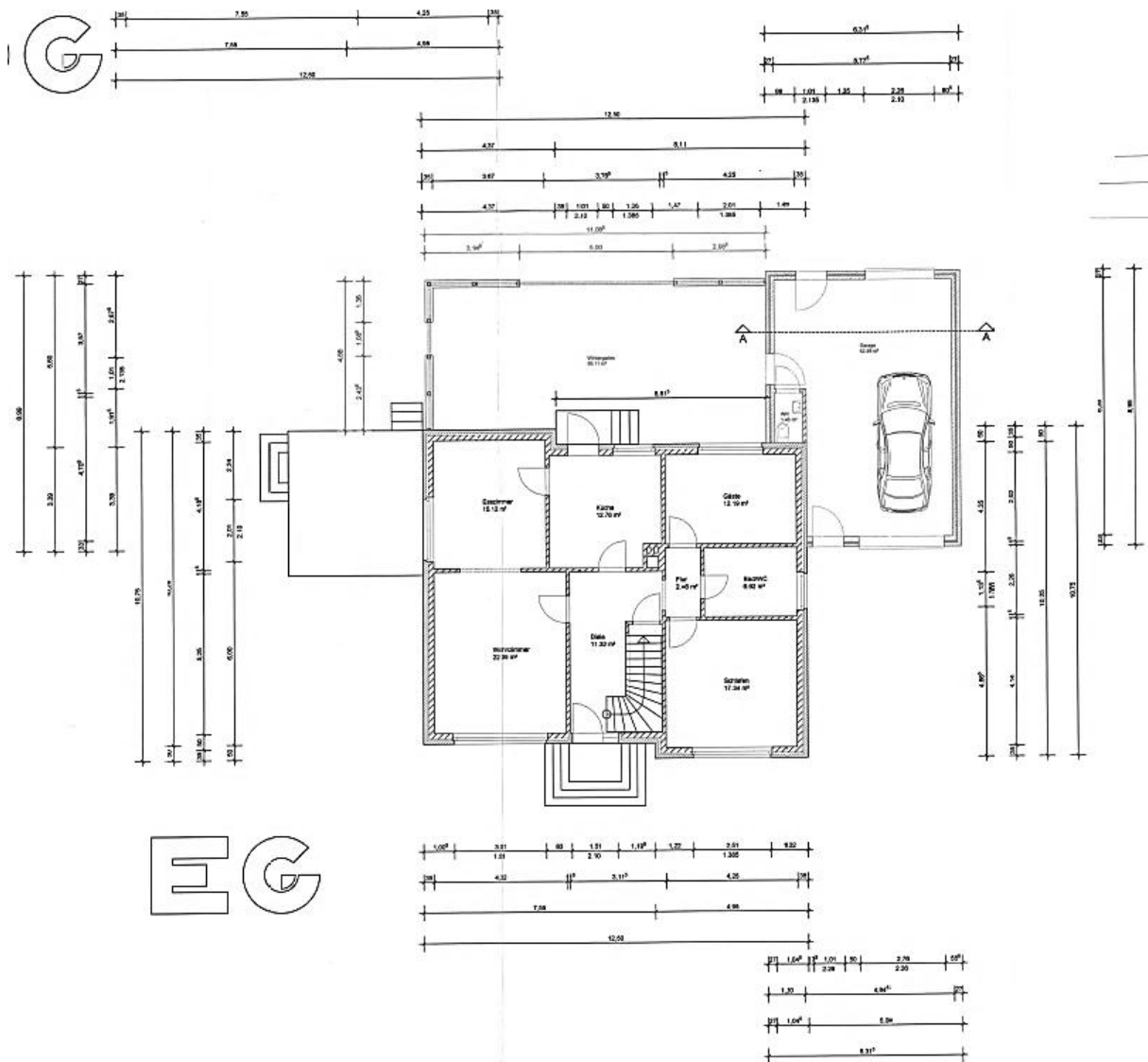
Grundriss Erdgeschoss
