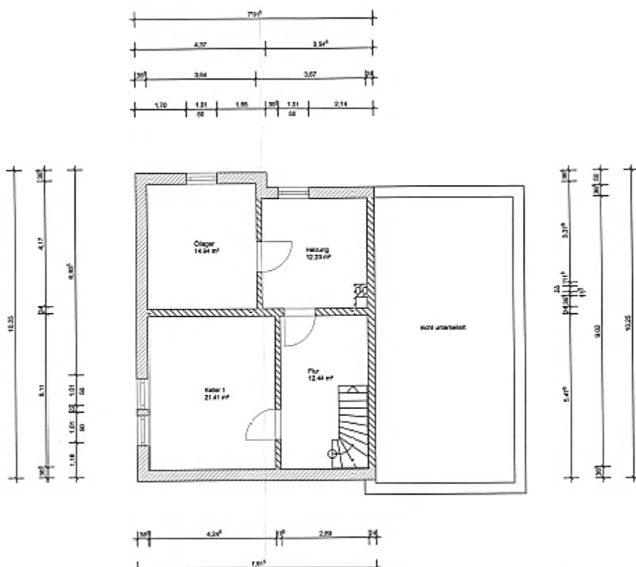
Grundriss Kellergeschoss
