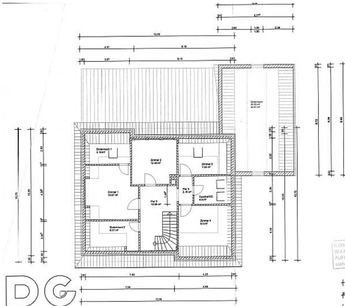
Grundriss Dachgeschoss
