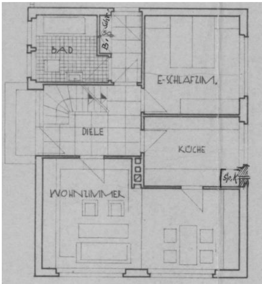
Auszug aus Bauakten (unmaßstäblich): Erdgeschoss
