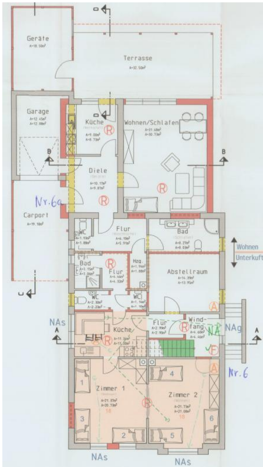
Grundrisszeichnung Erdgeschoss incl. Anbau
