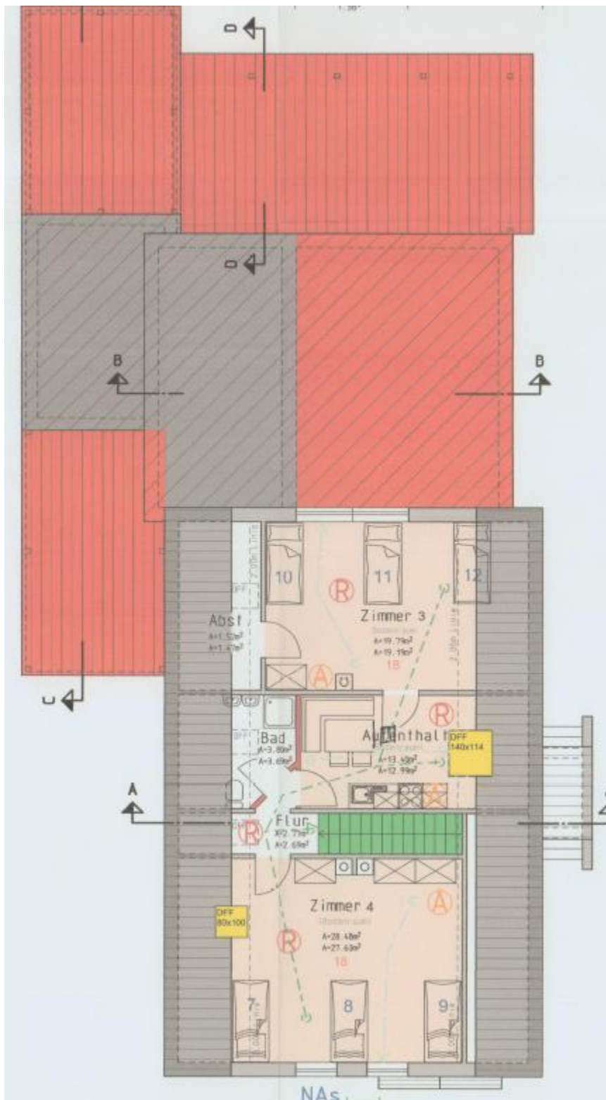
Grundriss Dachgeschoss
