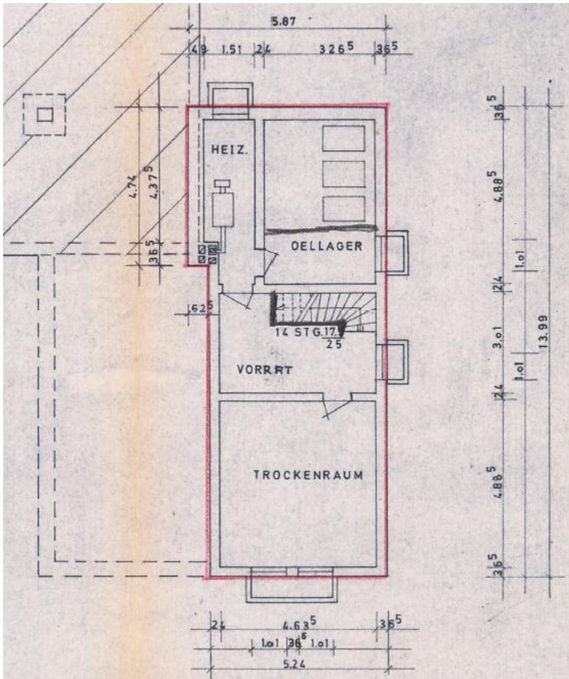
Grundriss Kellergeschoss
