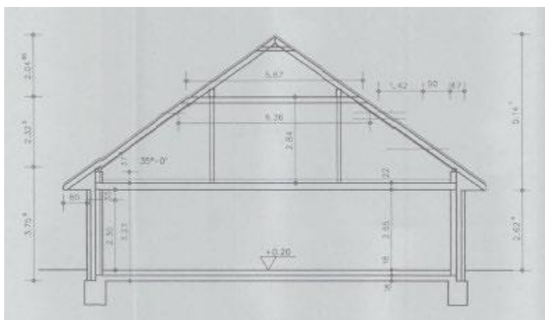
Gebäudeschnittzeichnung Wohnhaus
