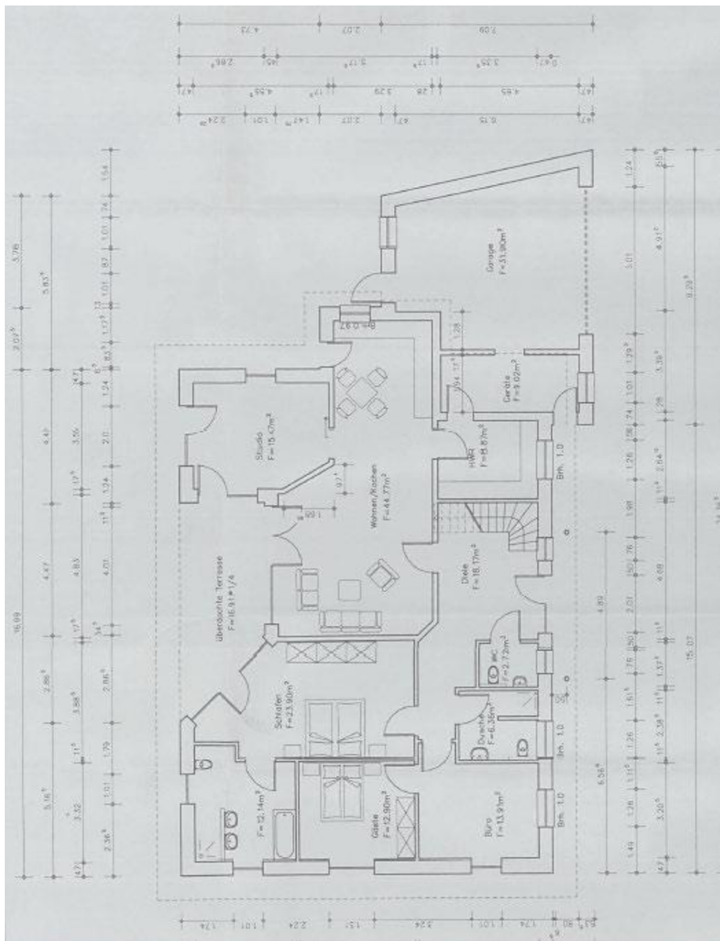
Grundriss EG
