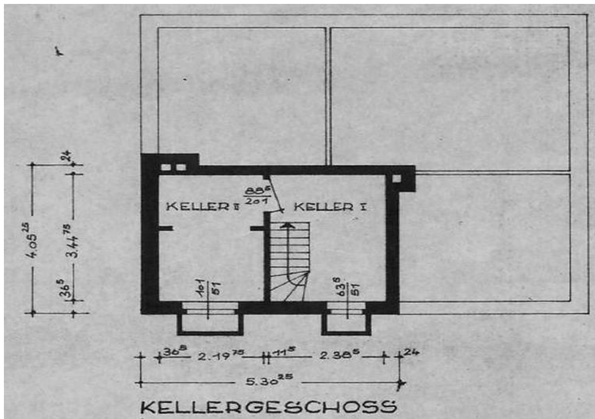
Grundriss Kellergeschoss
