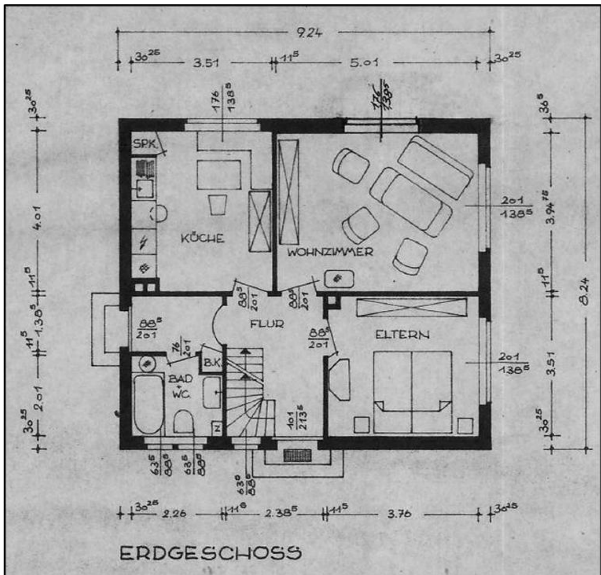
Grundriss Erdgeschoss
