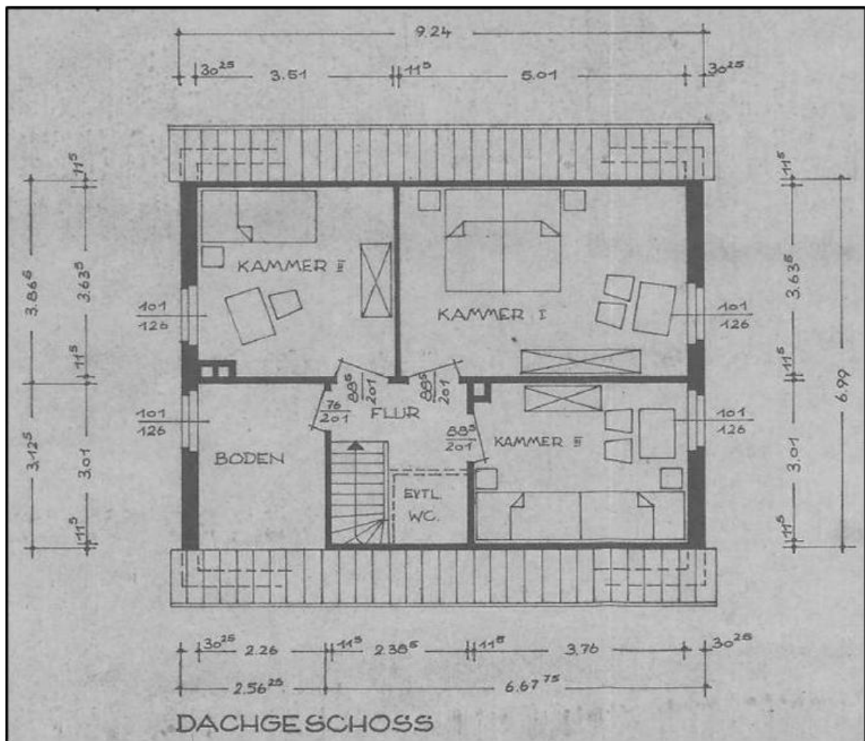
Grundriss Dachgeschoss
