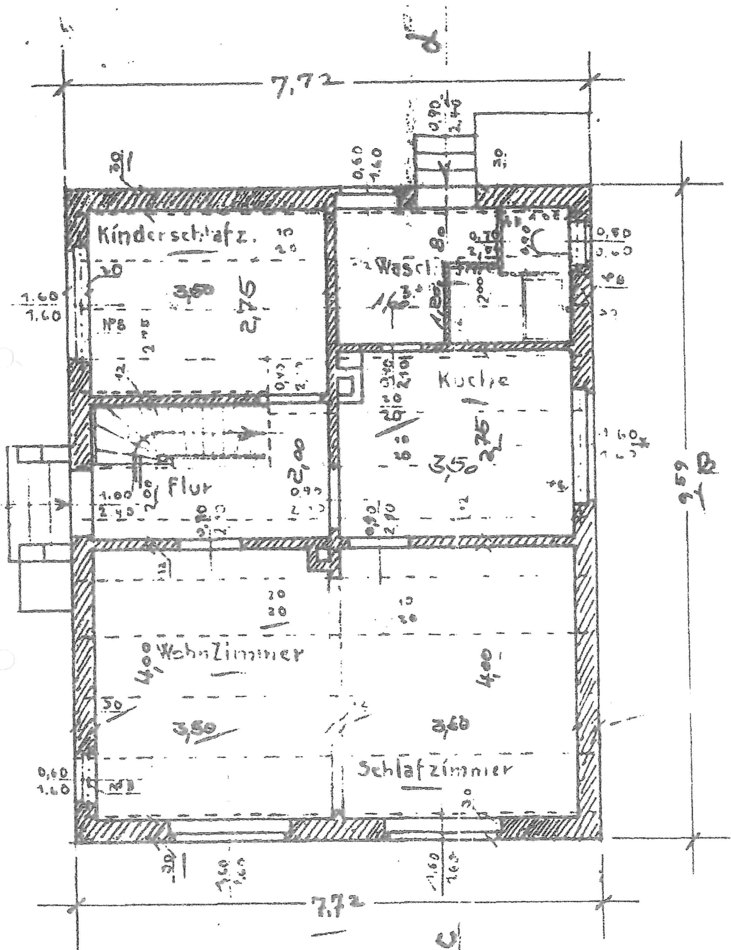
Erdgeschoßgrundriß.
