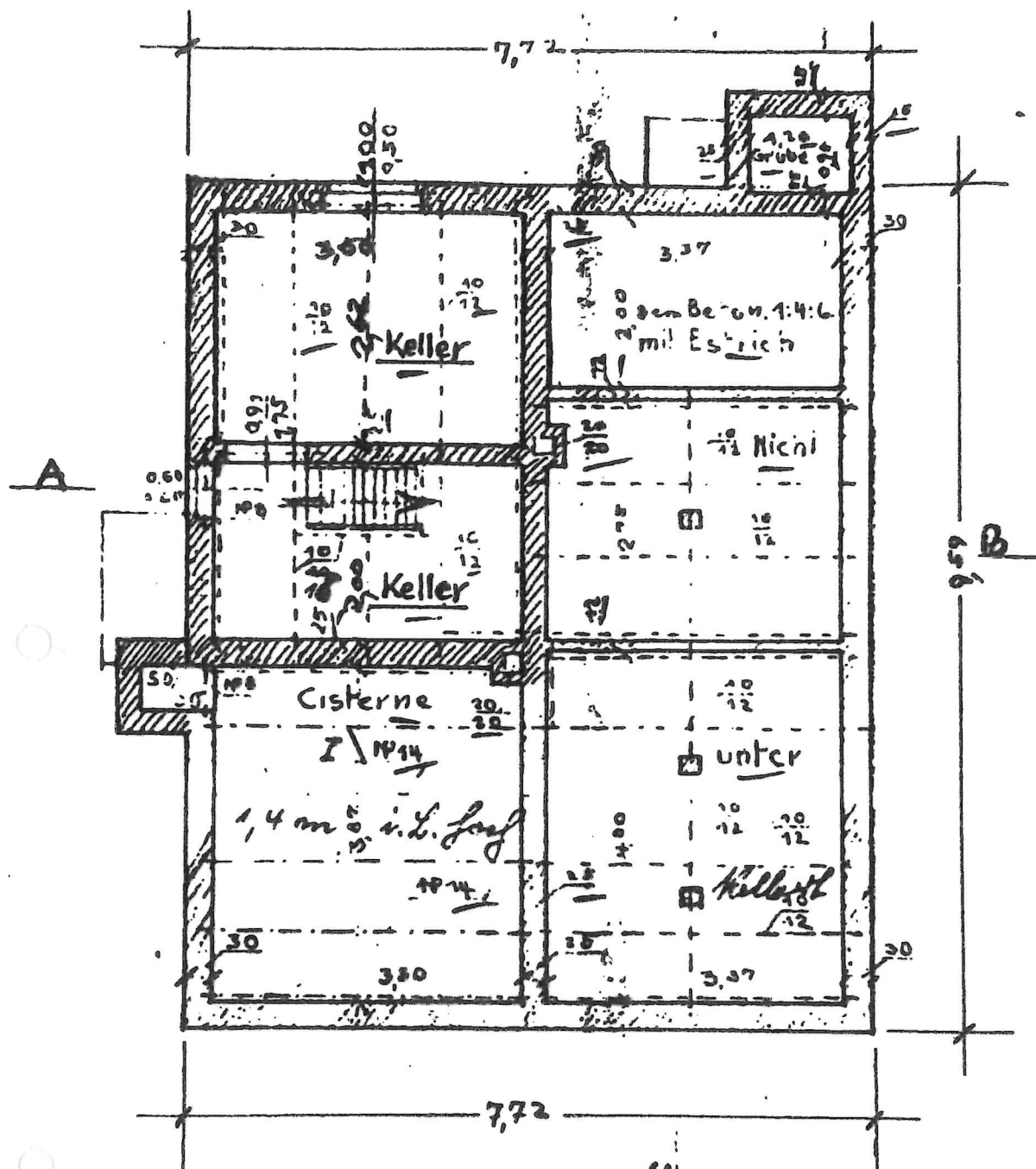
Keller geschoßgrundriß.
