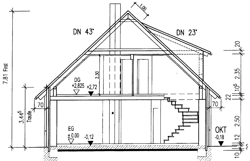
Schnitt
