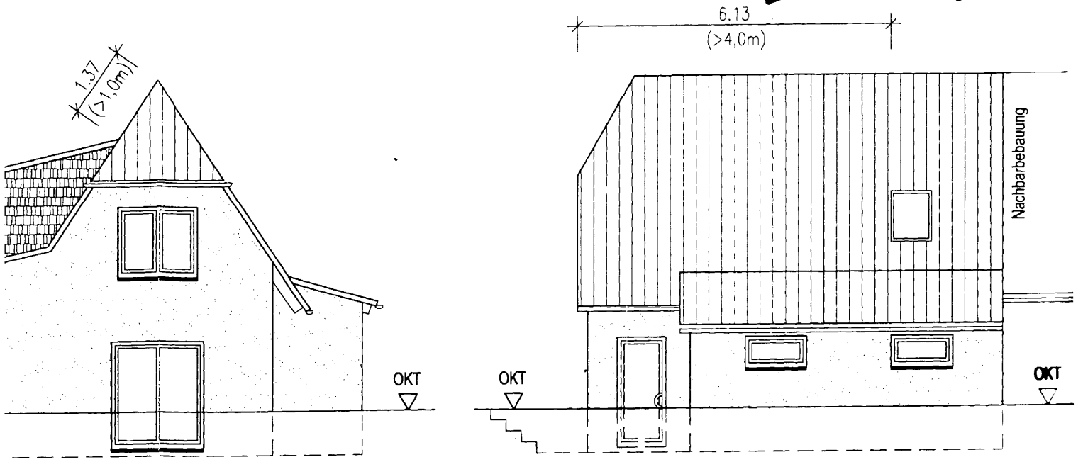
Nord-Ansicht
