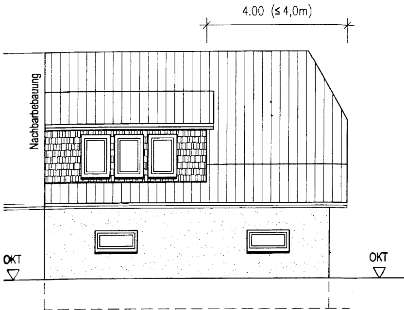
Süd-Ansicht
