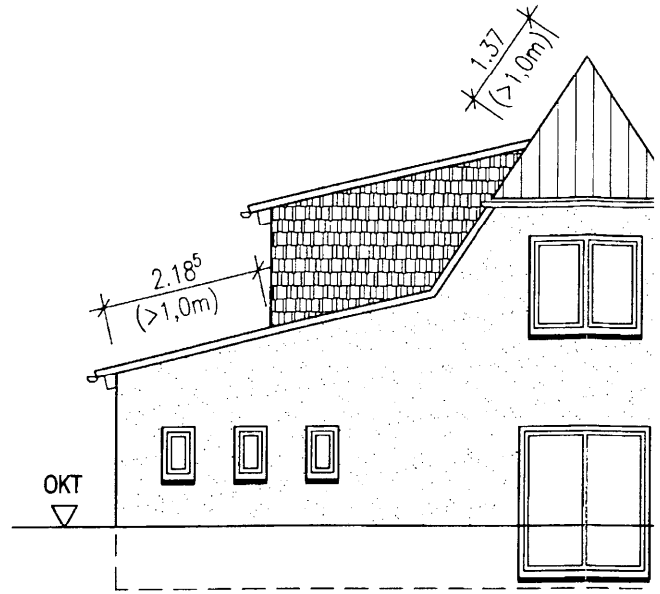
Ost-Ansicht
