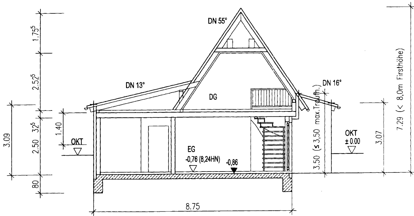
Schnitt B-B
