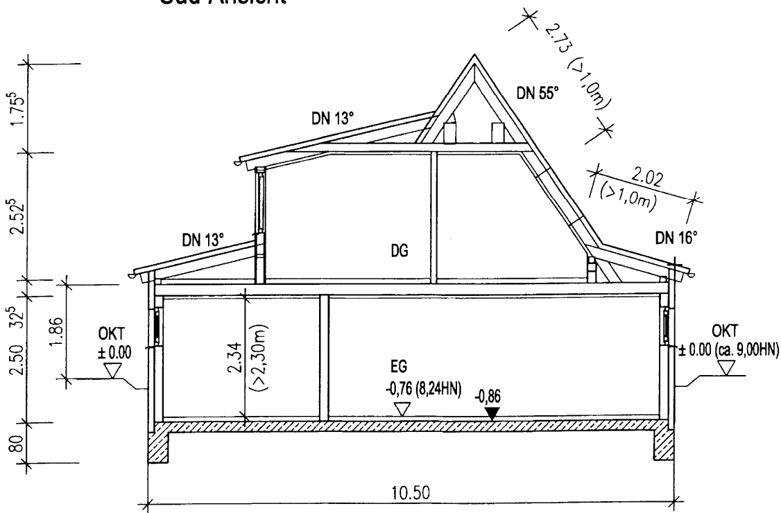
Schnitt A-A
