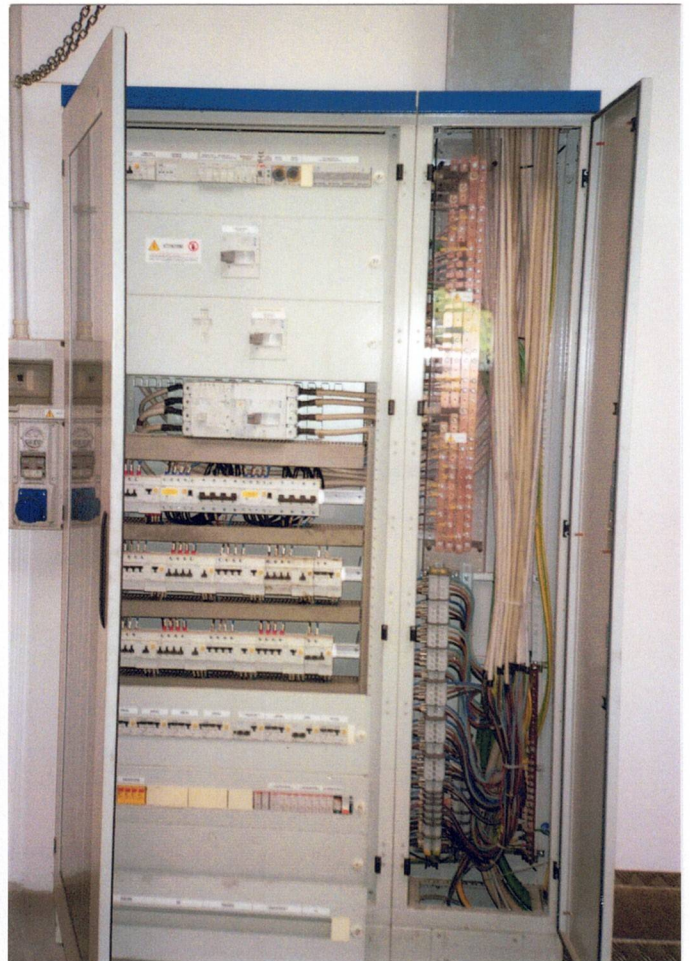
E-Verteilerschrank ostseitig
