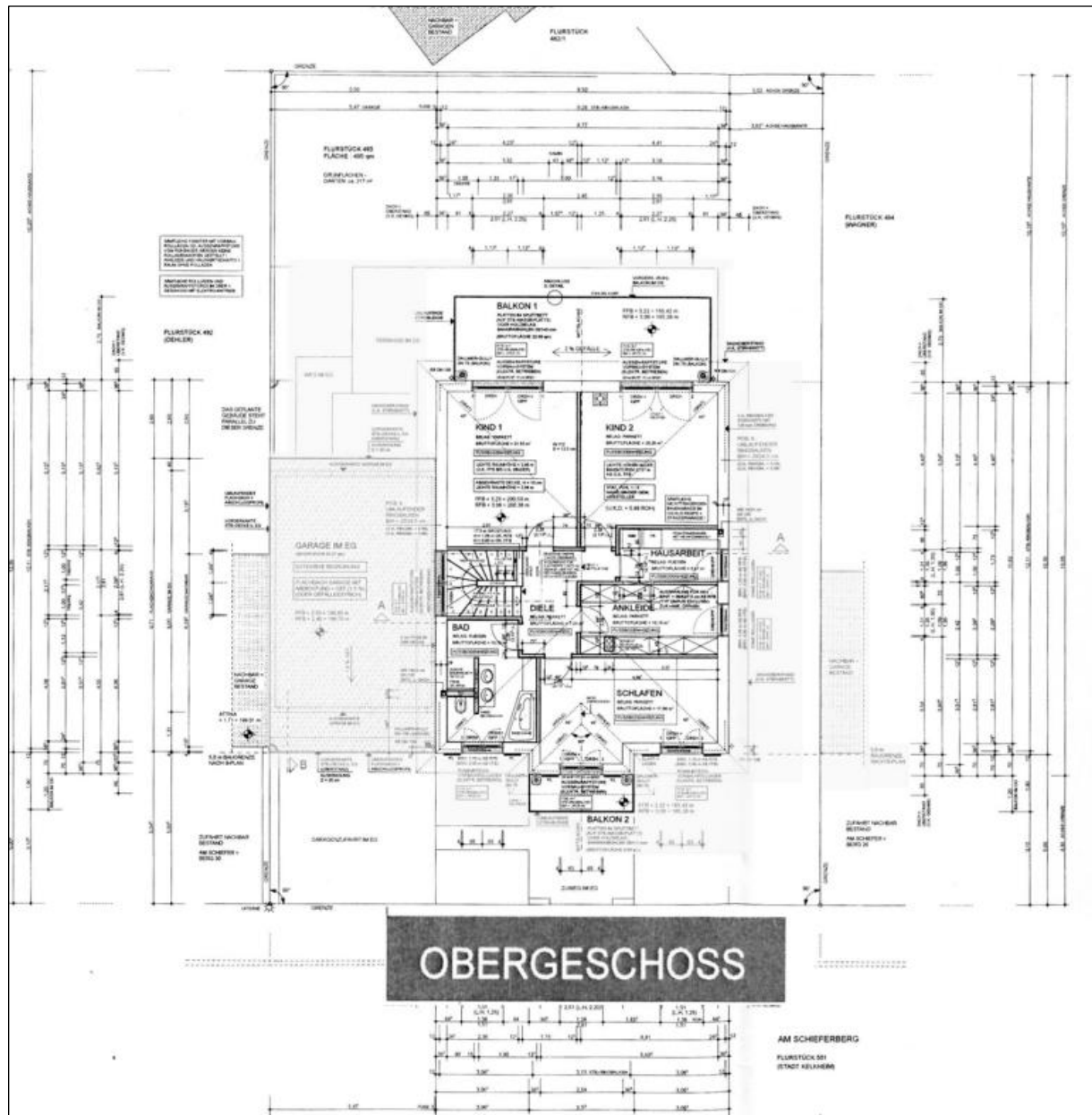
Obergeschoss
