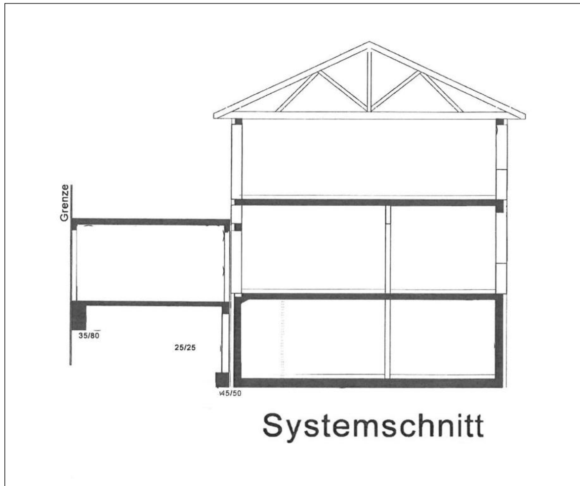
Schnitt
