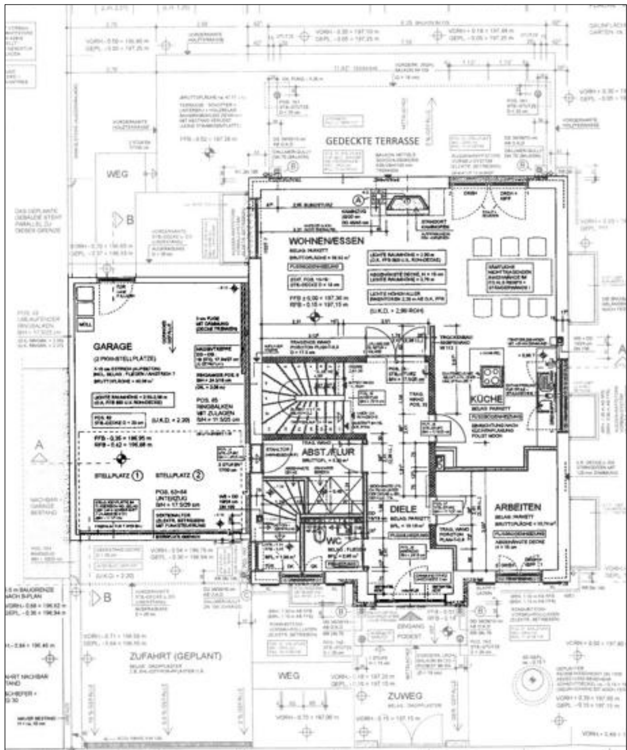
Erdgeschoss
