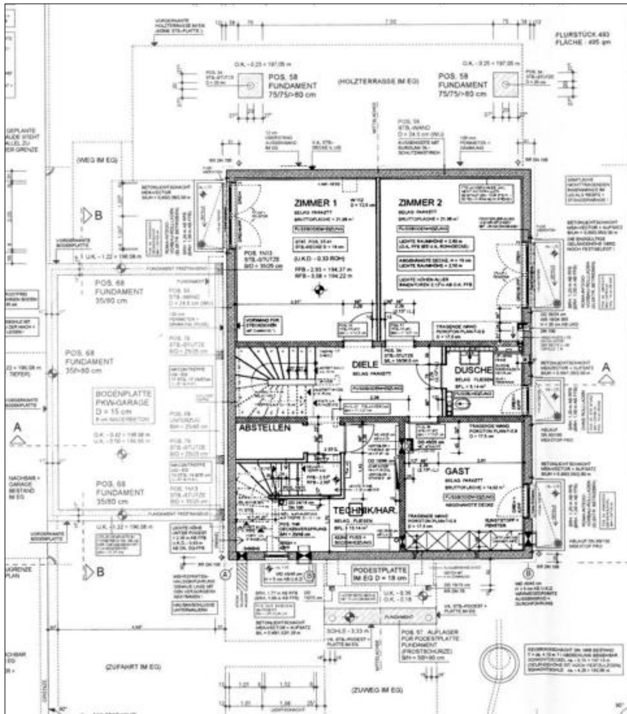
Kellergeschoss / Untergeschoss
