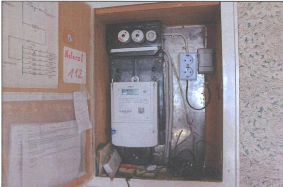
Bild C1 Beispiel Haustechnik
