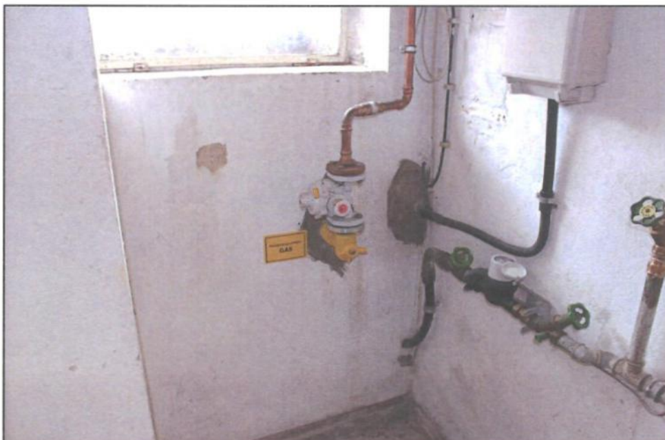
Bild C2 Beispiel Haustechnik
