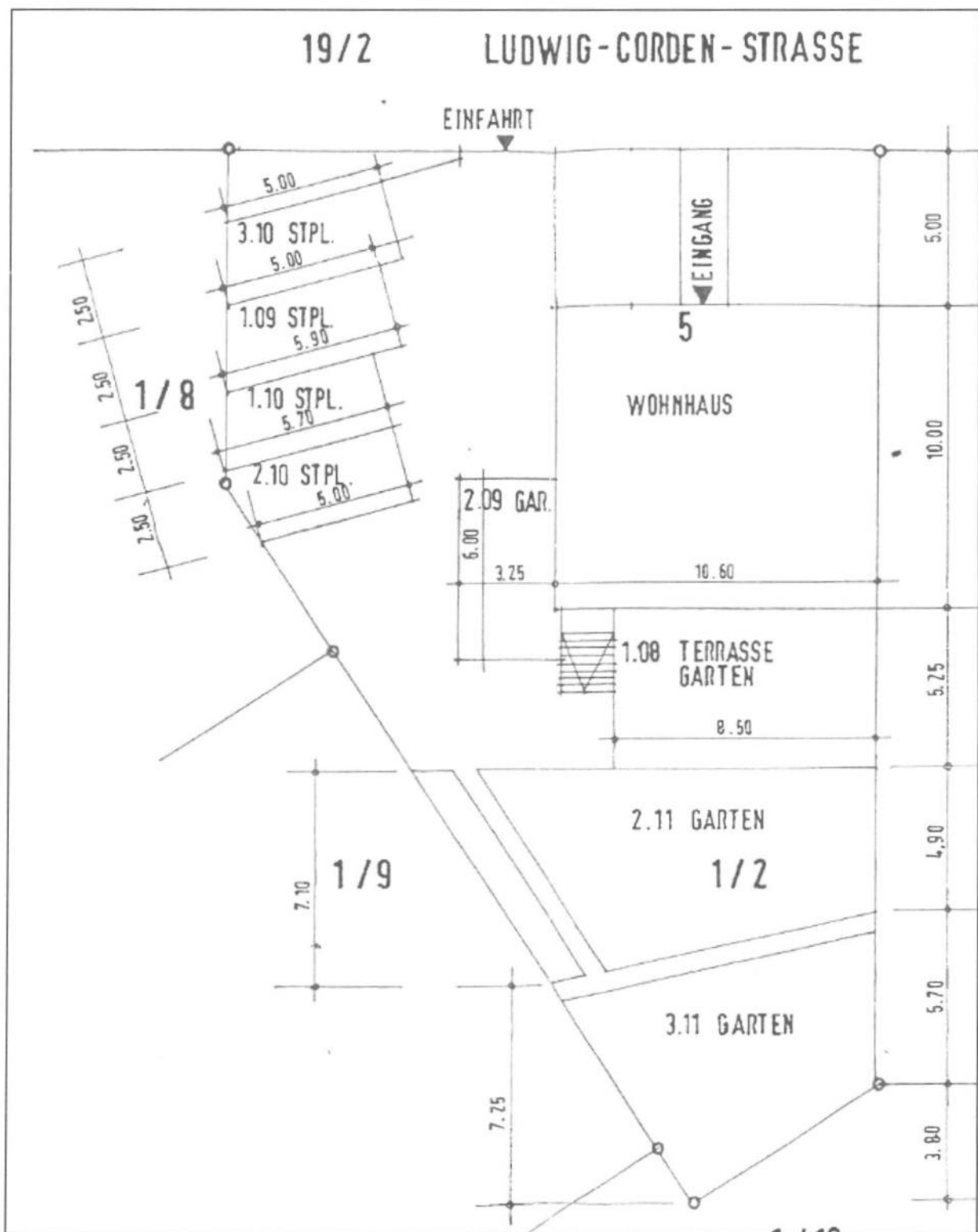
Freiflächenplan
