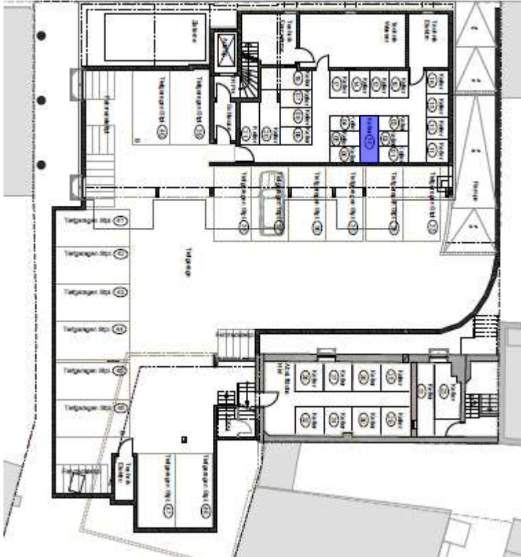
Übersicht UG mit Kellerabteil Nr. 18
