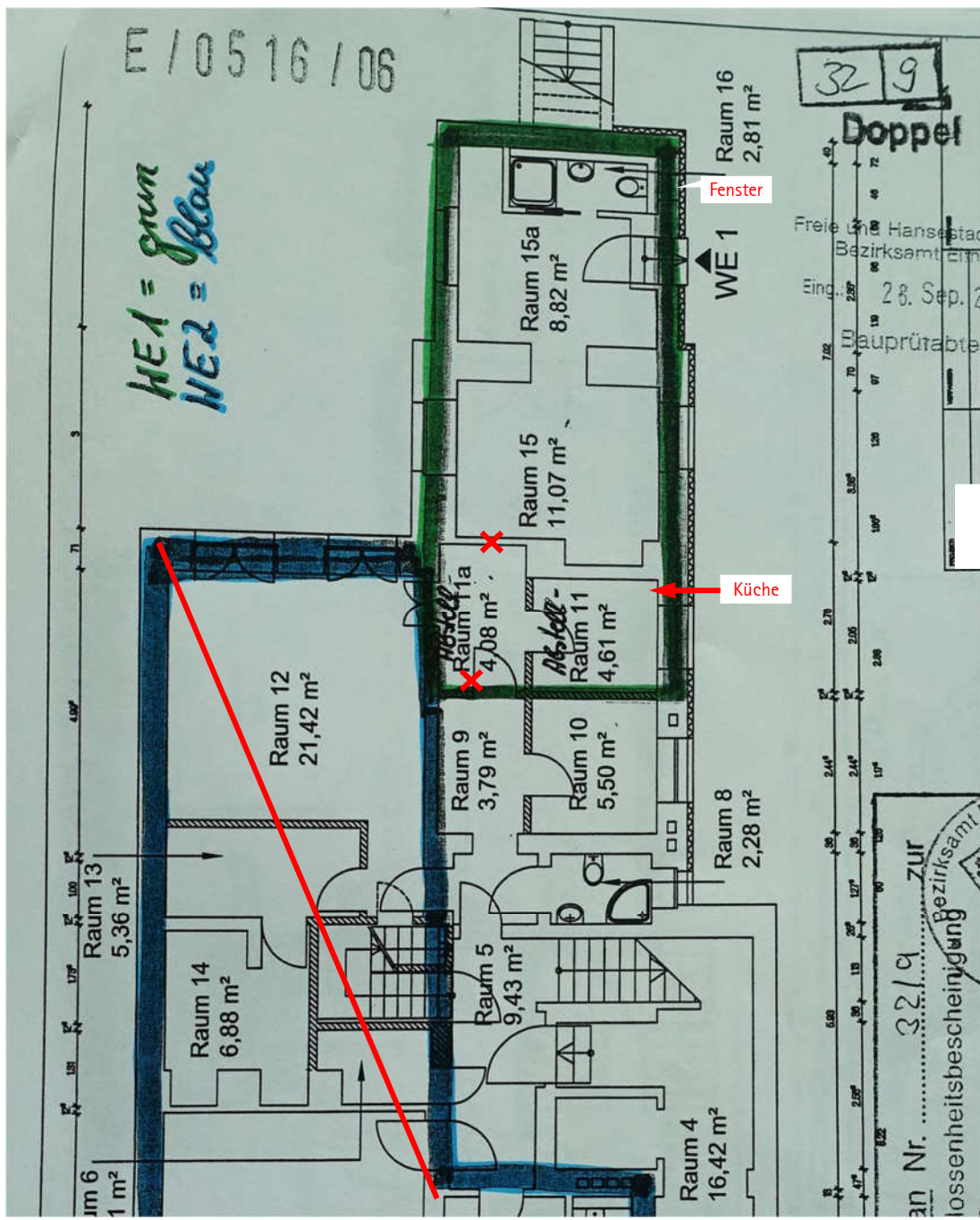
SE-Nr. WE 1 / Untergeschoss / Stand 2006 (Aufteilungsplan zur Teilungserklärung)
