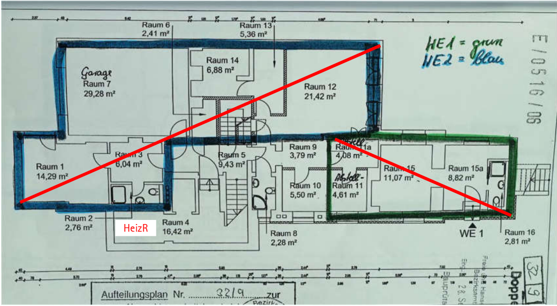
Querschnitt / Keller bzw. Souterrain / Stand 2006 (Aufteilungsplan zur Teilungserklärung) (Pläne hier ohne Maßstab / Norden unten / Quelle: Grundakte)
