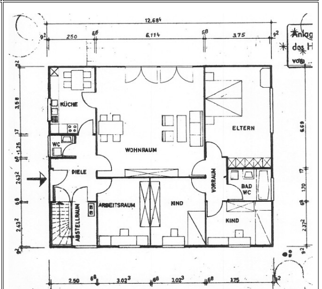
Erdgeschoss
