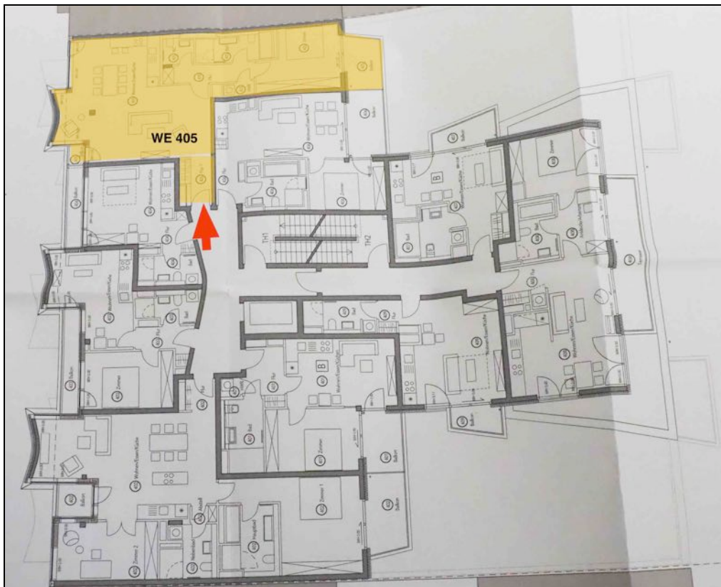
Grundriss 4. Obergeschoss
