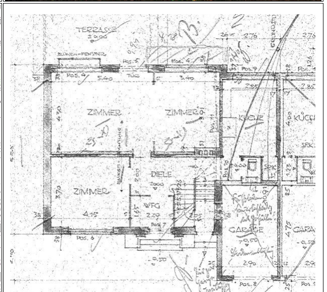
Erdgeschoss (Die Zeichnung stimmt teilweise nicht mit der Örtlichkeit überein.)
