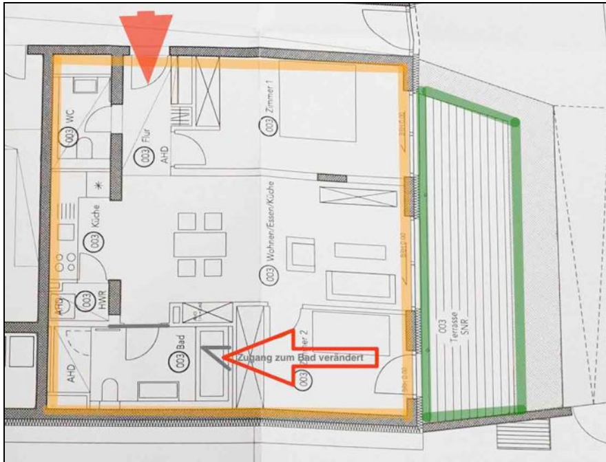
Grundriss Wohnung 003
