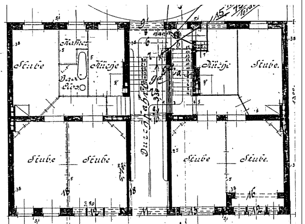
Vorderhaus Erdgeschoss
