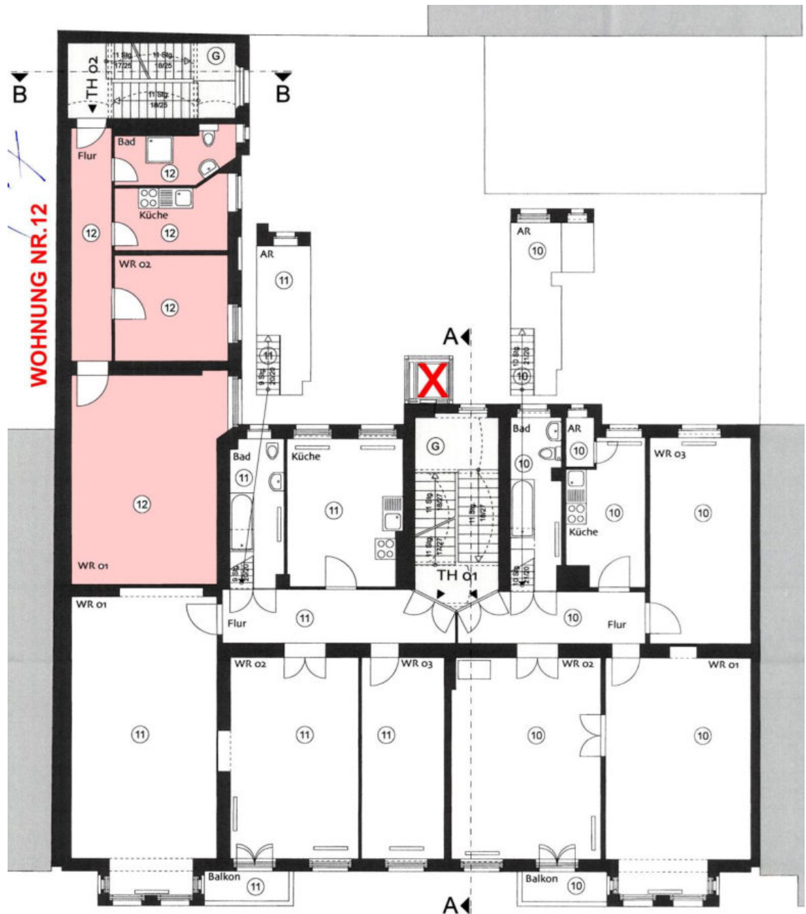
3. Obergeschoss
