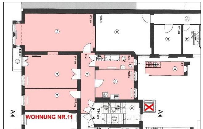
Grundriss 3. Obergeschoss
