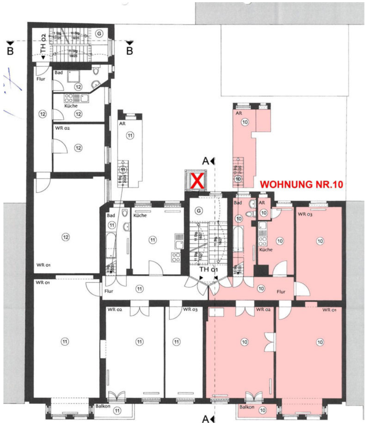
3. Obergeschoss
