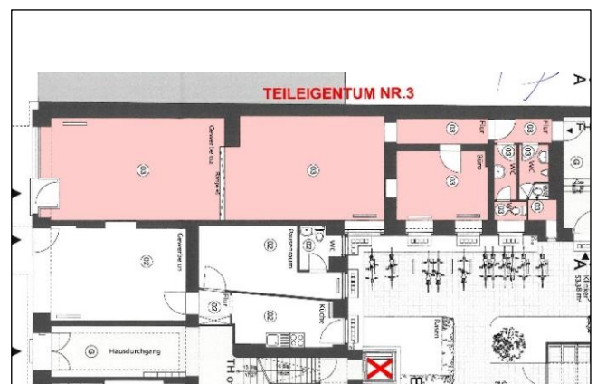
Grundriss Erdgeschoss
