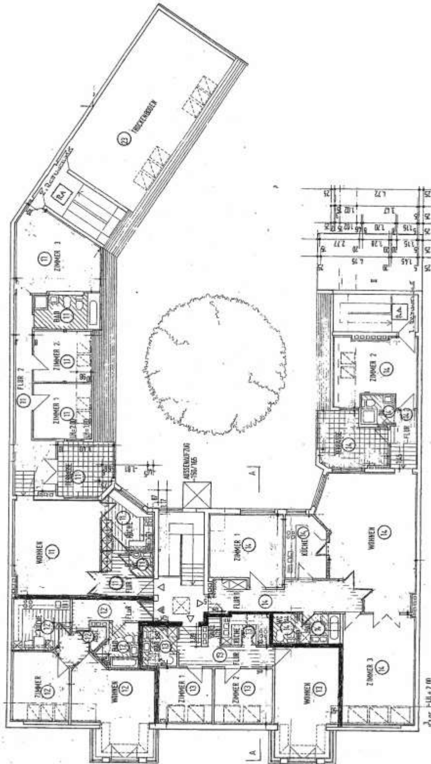
Aufteilungsplan Dachgeschoss
