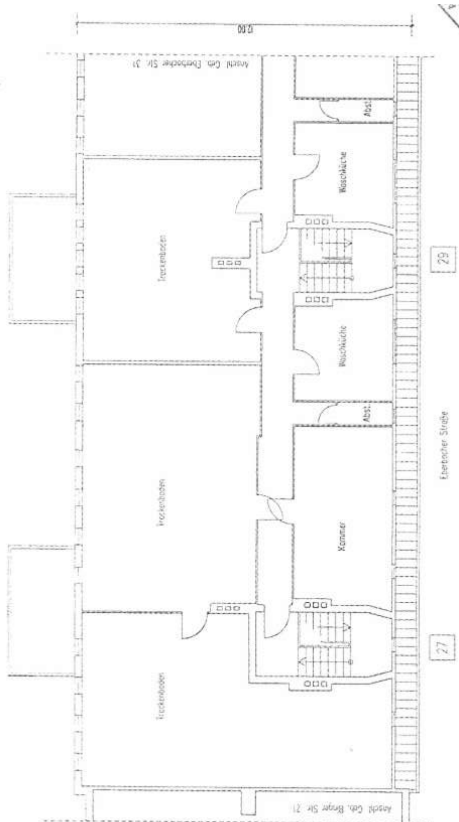
Grundriss Dachgeschoss, Gebäudeteile Eberbacher Str. 27 und 29
