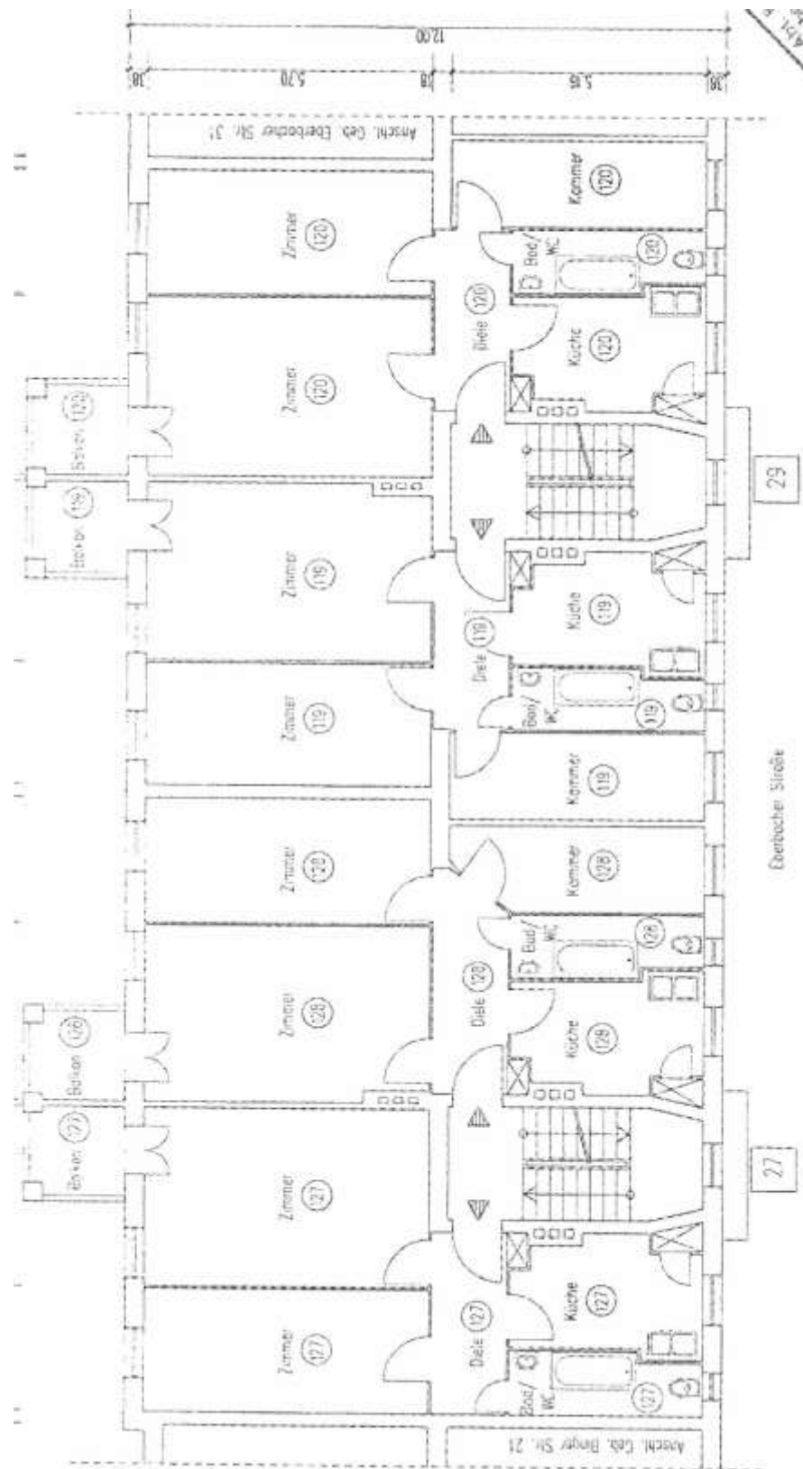
Aufteilungsplan 3. Obergeschoss, Gebäudeteile Eberbacher Str. 27 und 29
