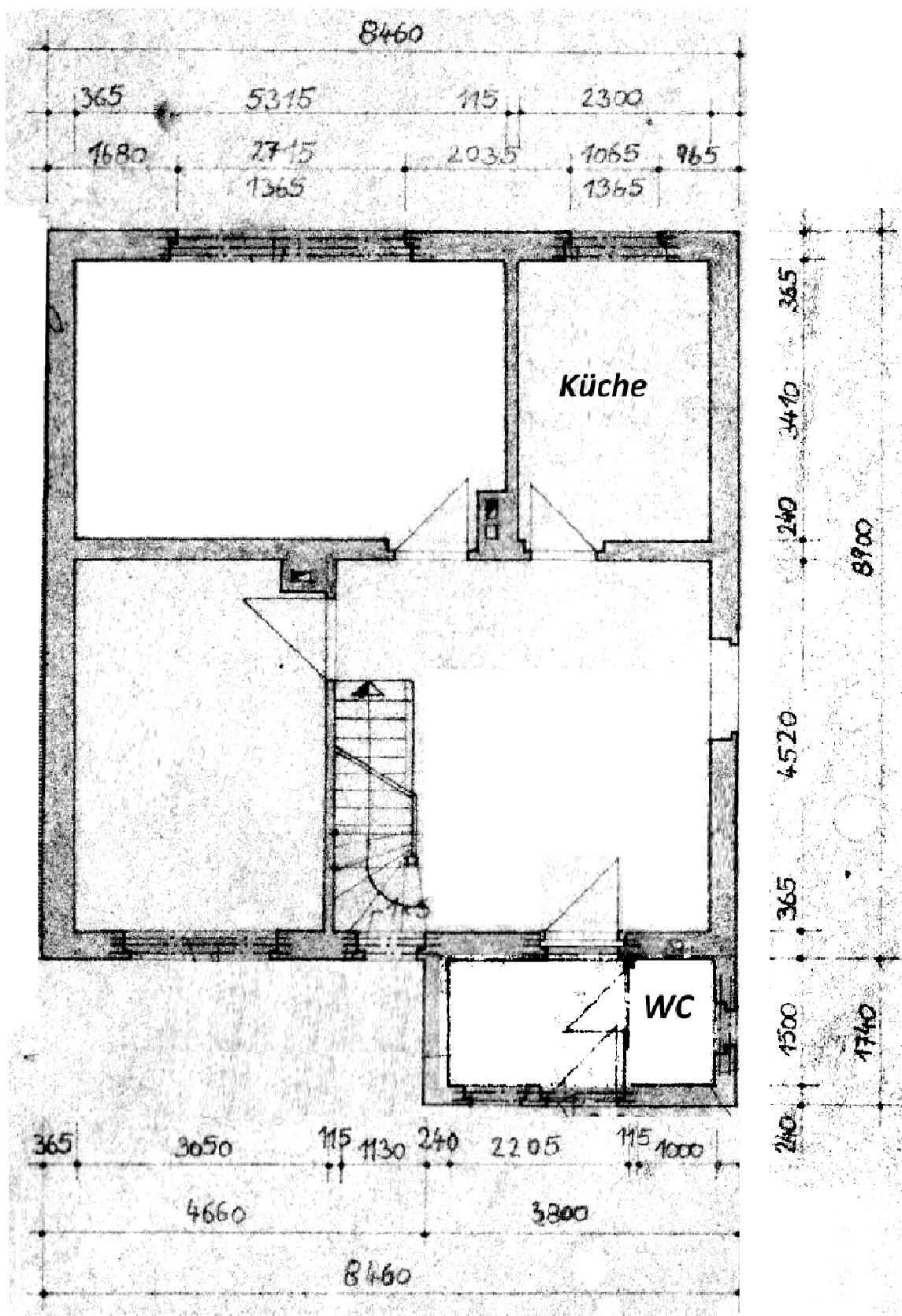
Ungefährer Grundriss vom EG (entnommen der Bauarchivakte) Leicht geändert durch den Gutachter entsprechend dem Bestand
