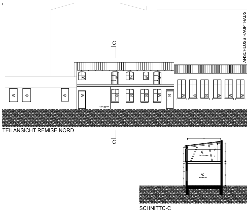
Abb. 9 Ansicht und Schnitt Remise
