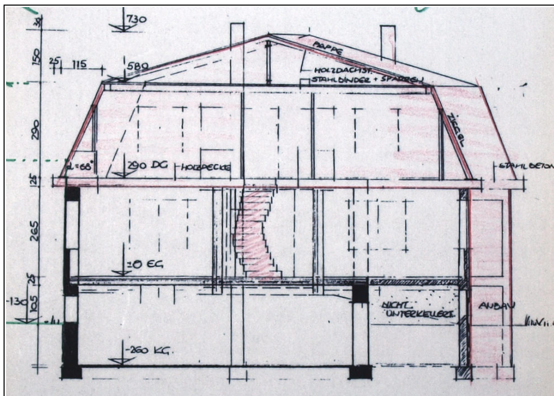
Abbildung 7: Schnittdarstellung
