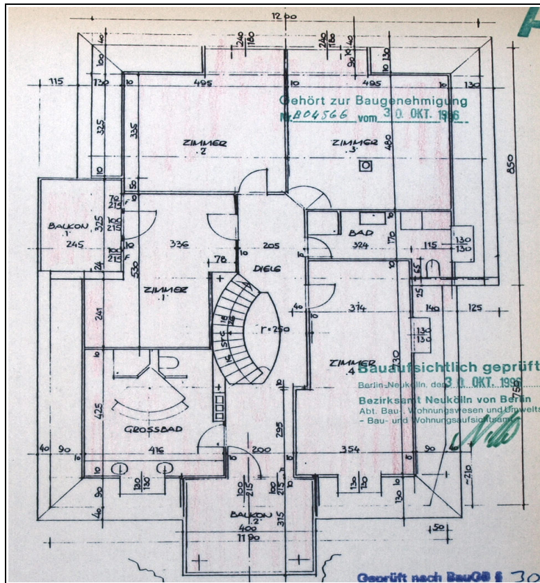
Abbildung 6: Grundriss Dachgeschoss
