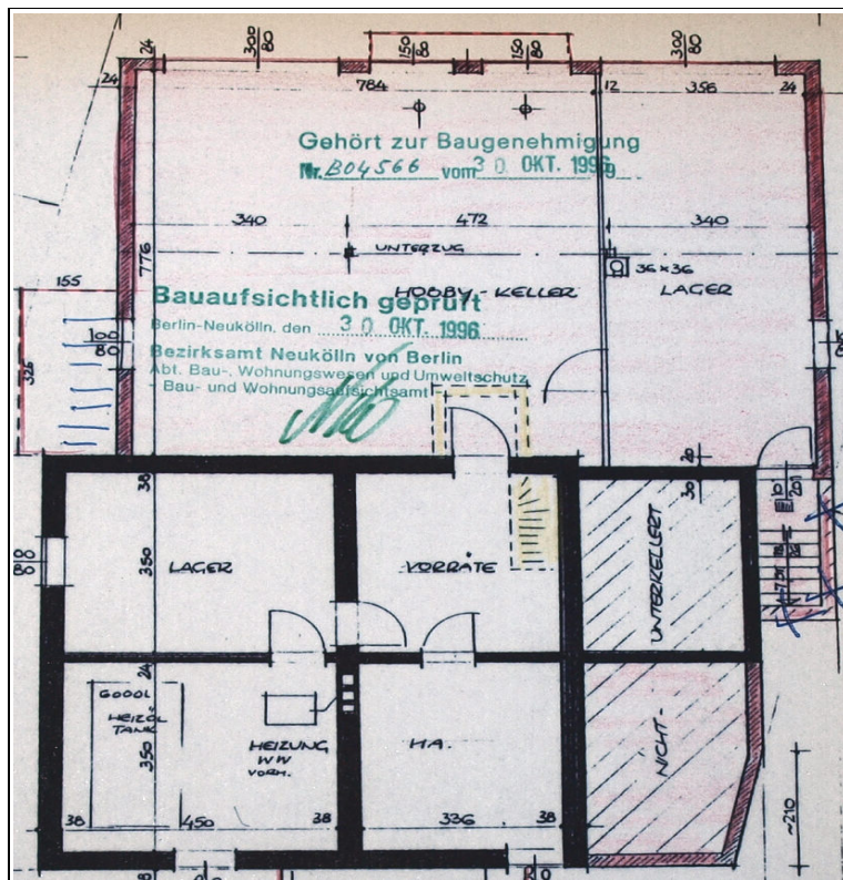
Abbildung 4: Grundriss Kellergeschoss
