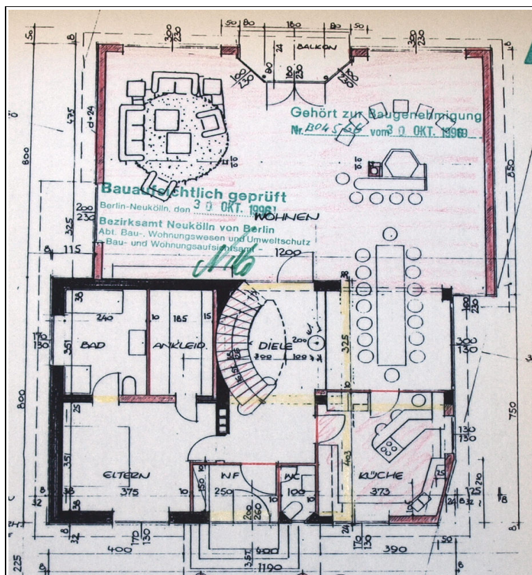
Abbildung 5: Grundriss Erdgeschoss
