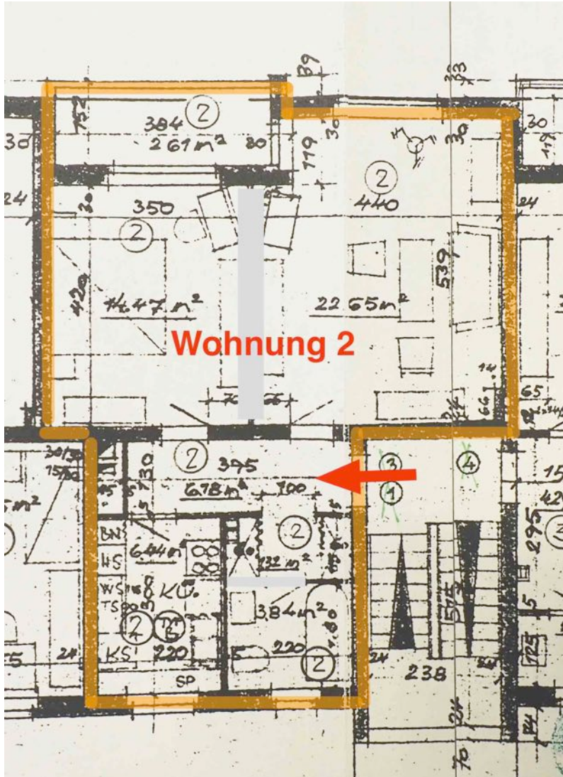
Grundriss Wohnung 2
