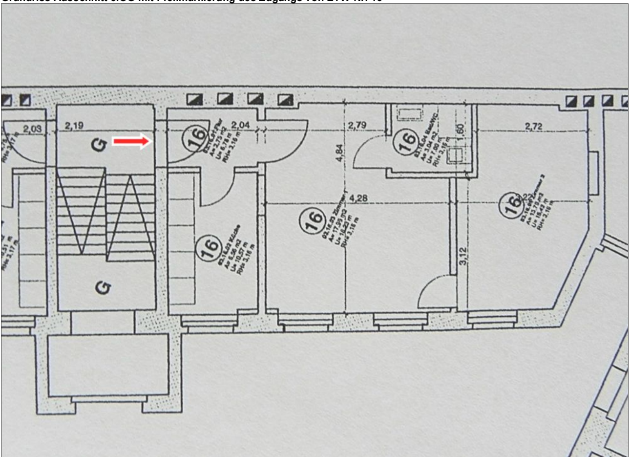
Grundriss Ausschnitt 3.OG mit Pfeilmarkierung des Zugangs von ETW-Nr. 16
