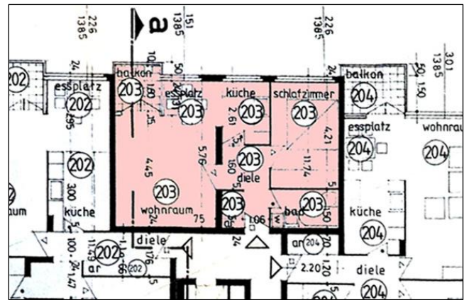
Grundriss 4. Obergeschoss
