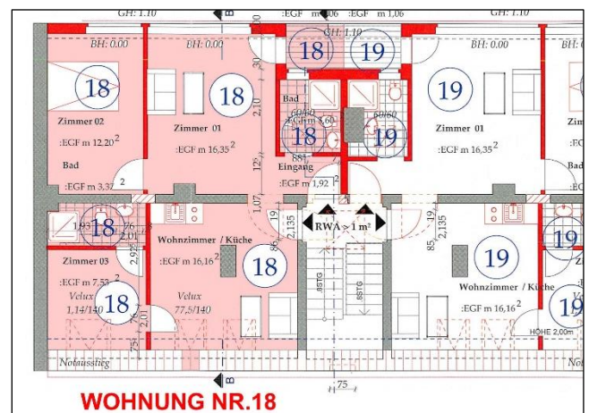
Grundriss Dachgeschoss (links)
